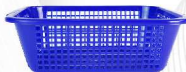
Canasta calada Susy no. 2 L: 345 An: 270 Al: 110 mm
