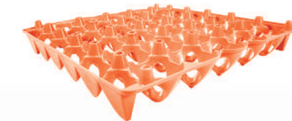
Charola de 30 cavidades L: 300 An: 300 Al: 55 mm
